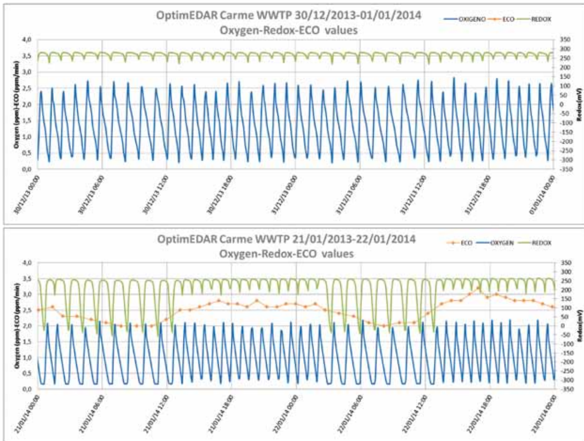
Figura 4. Evolución del oxígeno y del redox en el reactor biológico de la EDAR de Carme, antes (gráfico superior) y después (gráfico inferior) del control OptimEDAR.
